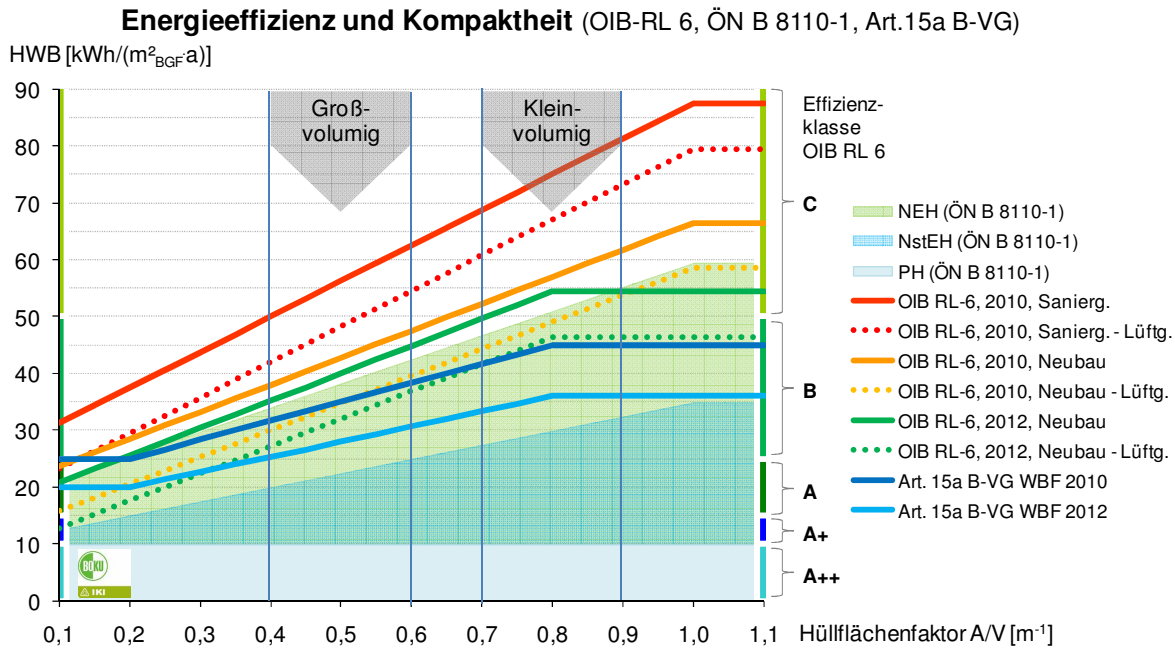
Abb.: Anforderungen an den spezifischen Heizwärmebedarf in Abhängigkeit des Hüllflächenfaktors (Oberflächen-Volumen-Verhältnis) gemäß OIB Richtlinie 6, ÖN B 8110-1 und §15a-Vereinbarung B-VG
