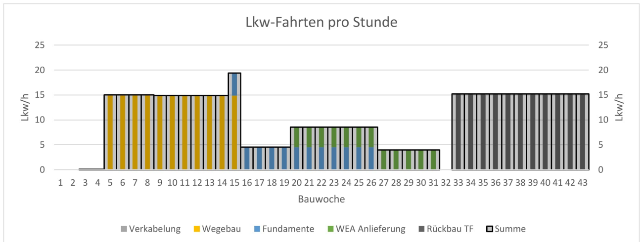
Abbildung 9: Anzahl der Lkw-Fahrten pro Stunde über die Bauzeit
