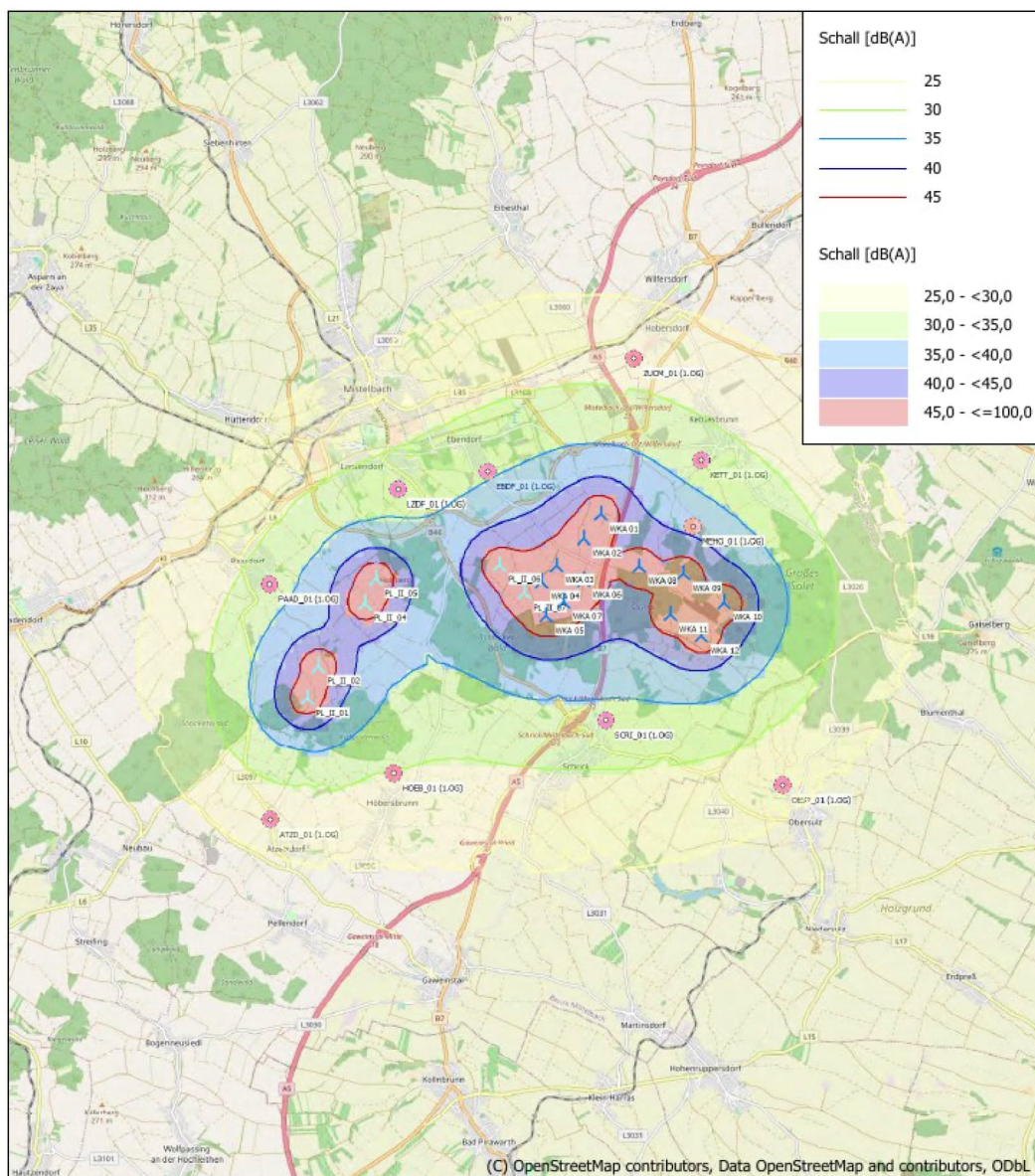
Abbildung 2: Rasterlärmkarte, betriebskausale Immissionen, Wirkfaktorenbericht
