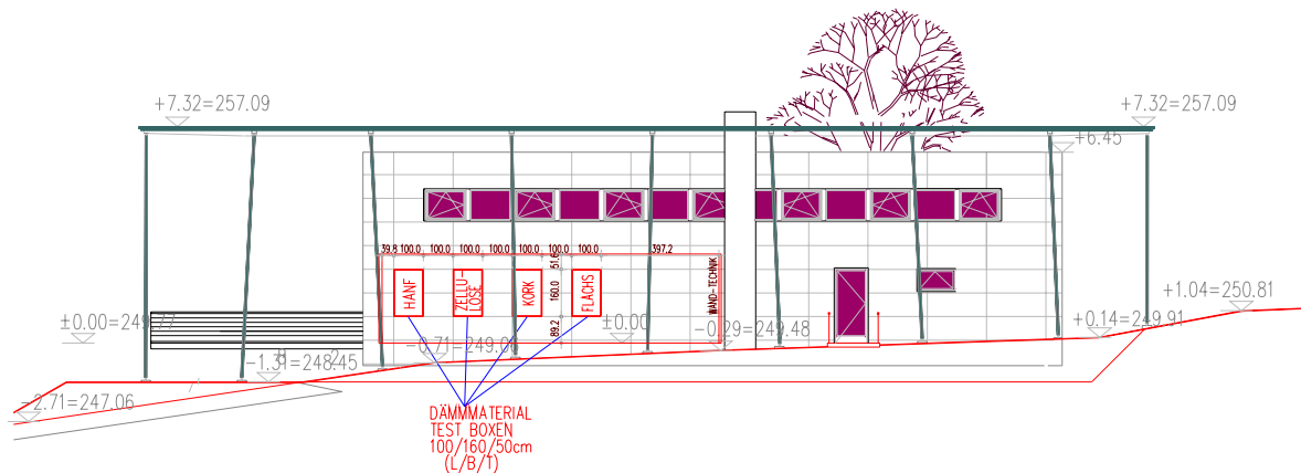
Abbildung 27: Lage der Testboxen an der Nordwand
