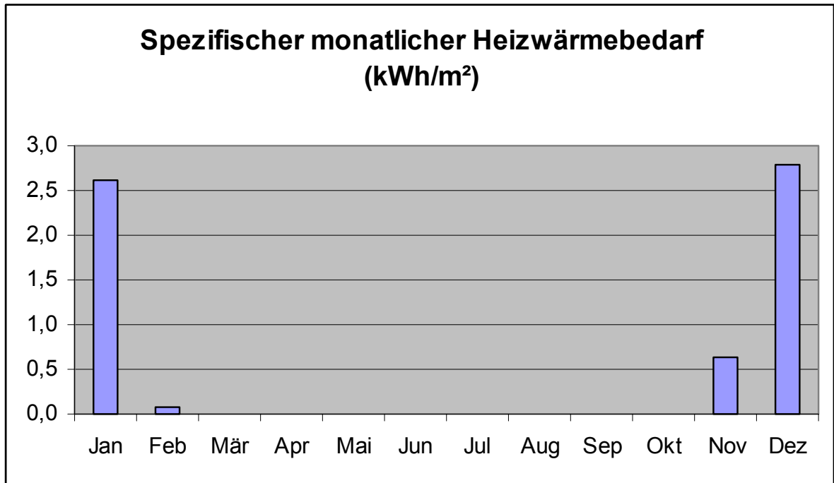
Grafik 8: Spezifischer monatlicher Heizwärmebedarf
