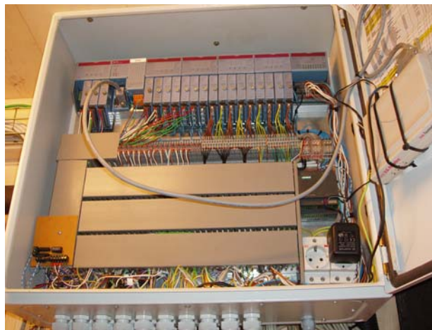
Abbildung 30: Loggersystem AEE INTEC
