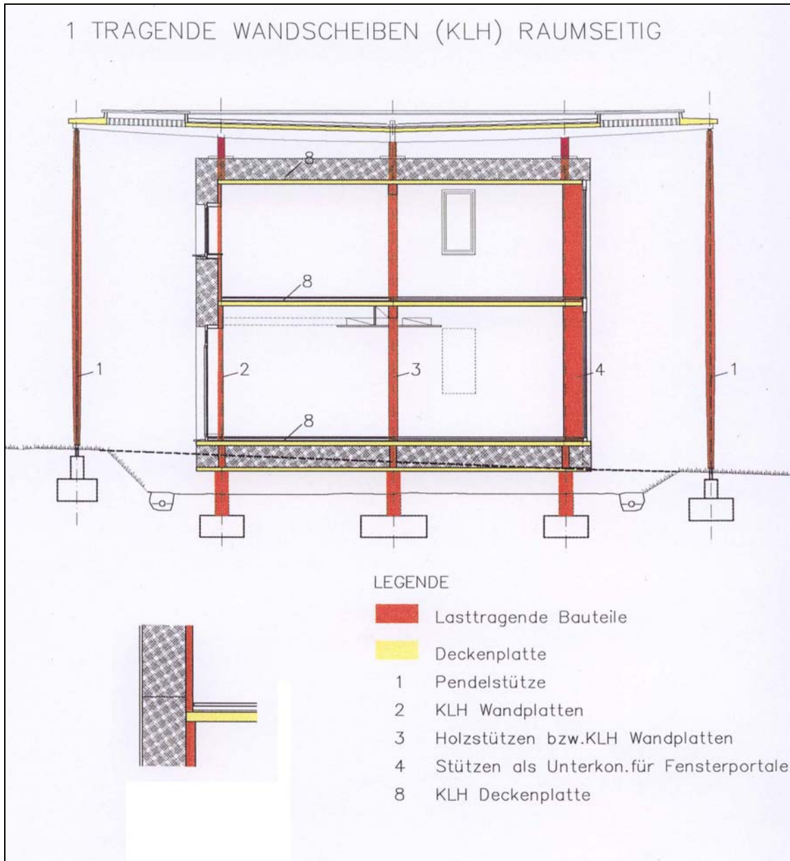
Grafik 5: Tragende Wandscheiben (KLH) raumseitig
