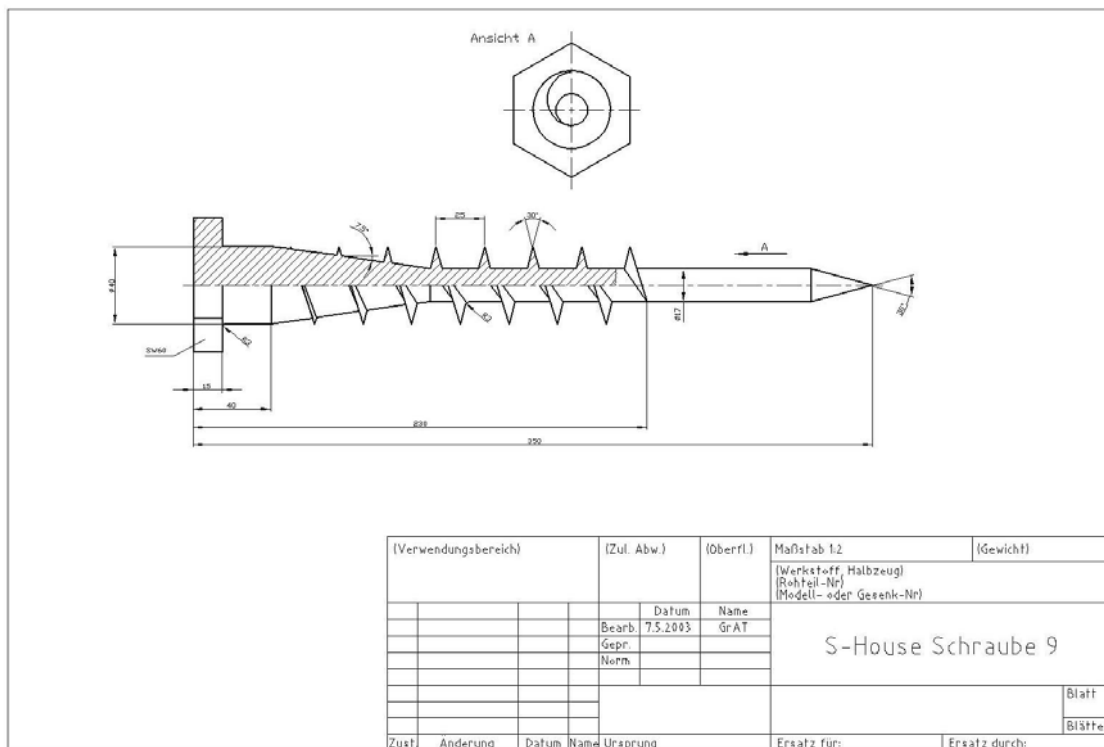
Grafik 2: TREEPLAST Schraube als Befestigungselement im S-HOUSE
