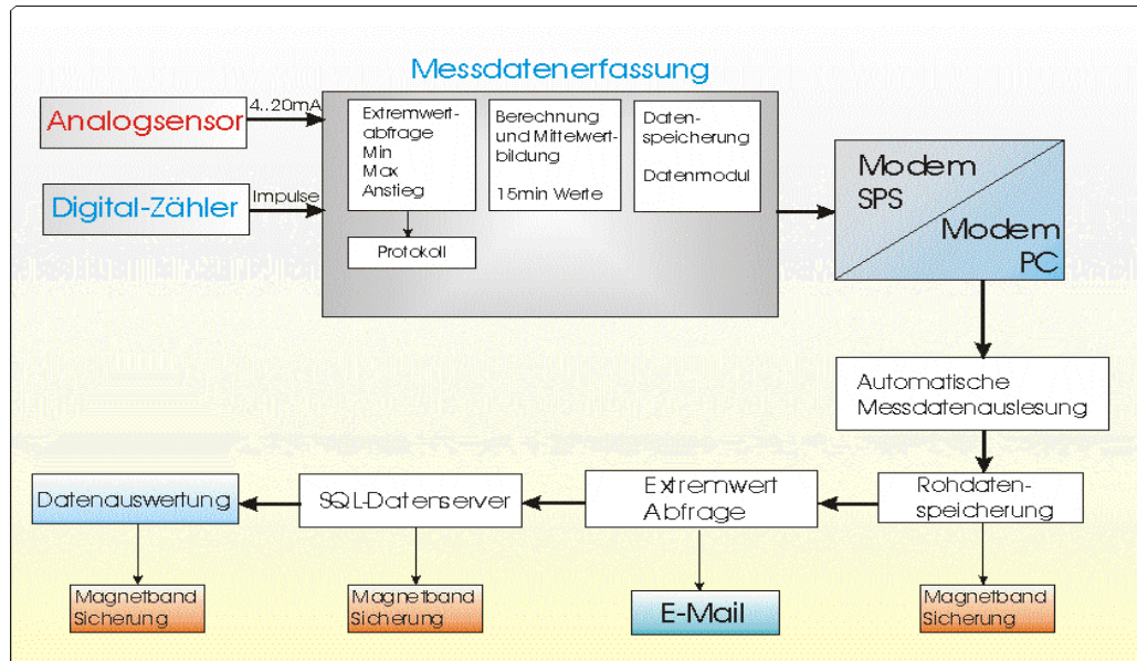
Abbildung 31: Schema der Datenaufzeichnung und Weiterverarbeitung
