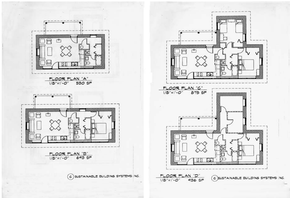
Grafik 1: Grundrisse von Strohhäusern für sozial Bedürftige, Planung: Alfred von Bachmaier
