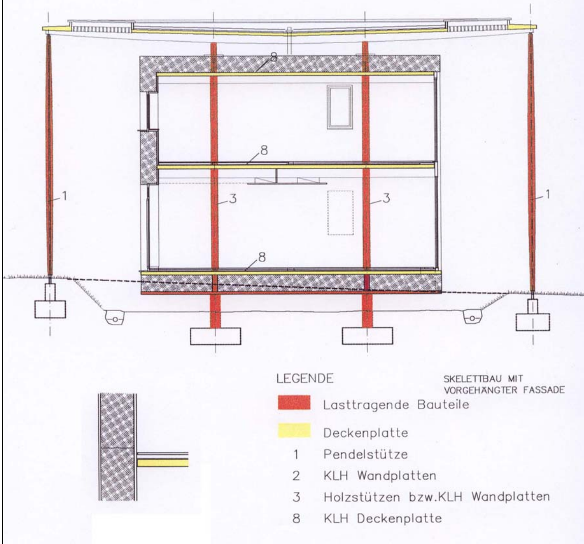
Grafik 6: Skelettbau mit Strohballenaussenwand
