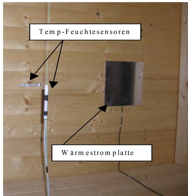
Abbildung 28: Anordnung der Messfühler in den Testboxen
